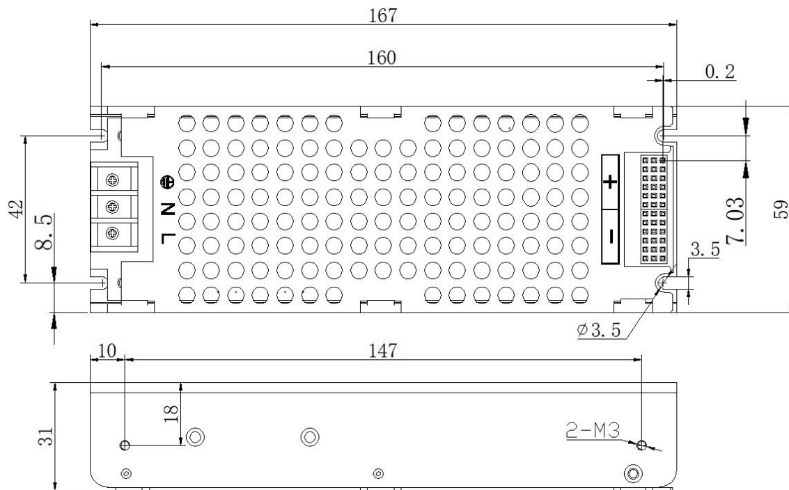
c. CL-AS11-200-5D 外形尺寸
