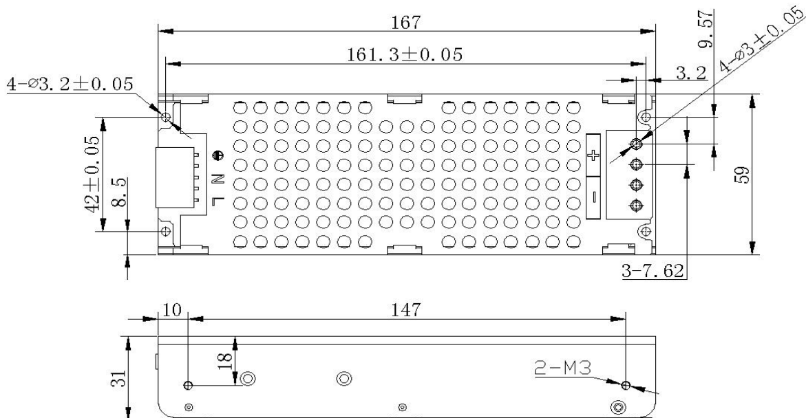
b. CL-AS11-200-5B 外形尺寸
