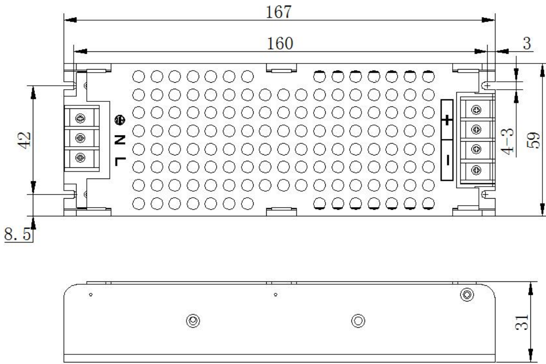
c. CL-AS11-200-5D 外形尺寸
