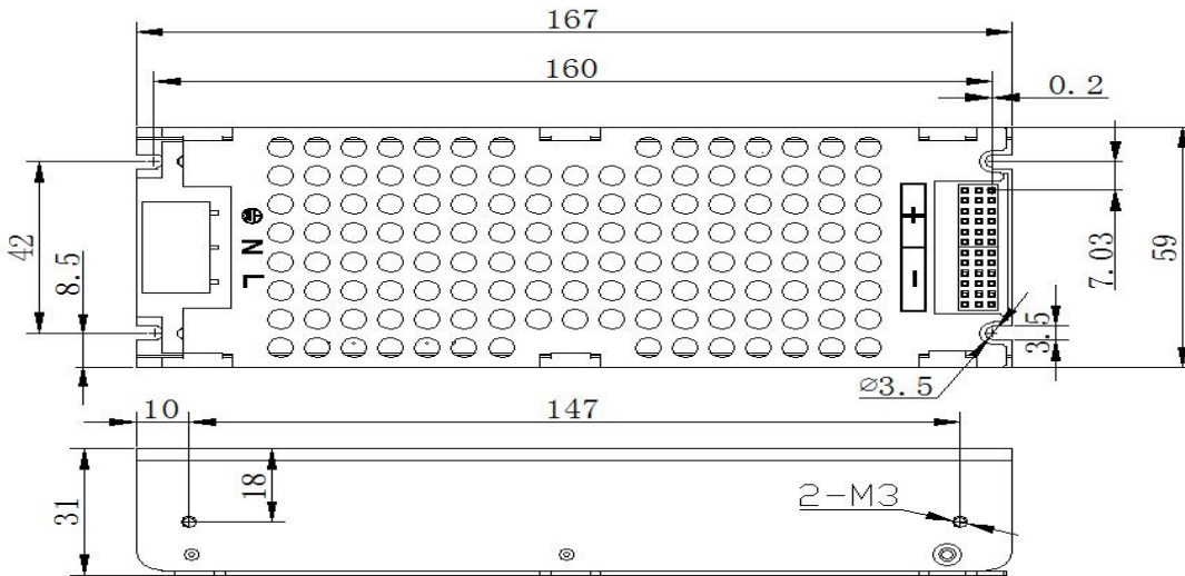
b. CL-AS11-200-5B 外形尺寸
